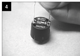
Draht anschließen (12V-/AC) an der LED-Einheit.
