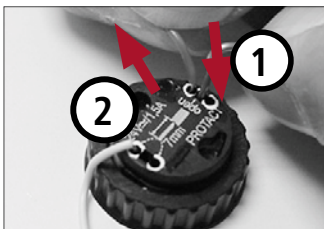
Bei starrem Draht direkt anschließen. Bei flexiblem Draht zuerst mit beiliegendem Hilfswerkzeug, in der Mitte entriegeln.
