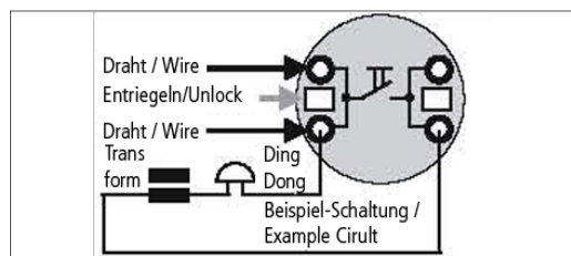
Draht anschließen (12V-/AC) an der LED-Einheit.
