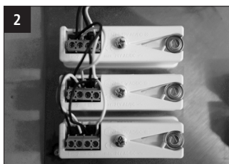
2 Anschluss Klingel max. 24V AC/DC. Anschluss Beleuchtung max. 12V AC/DC.
