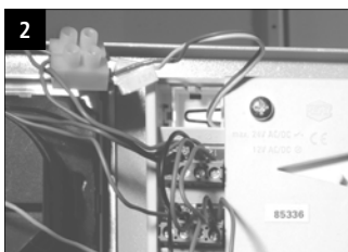
Anschluss Beleuchtung max. 12V AC/DC
